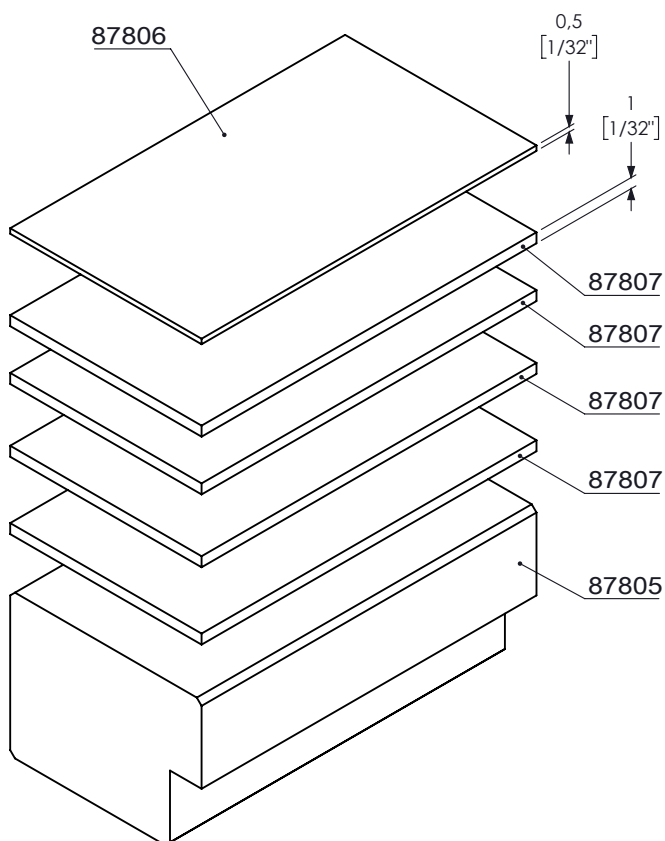
Kit distanziali vetro Kit glass spacer Kit distanciales para vidrio
