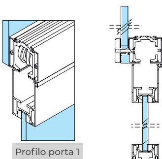
Profilo porta 1
