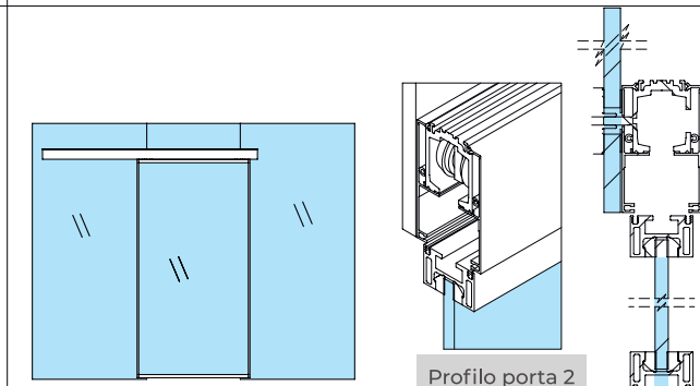
Profilo porta 2
