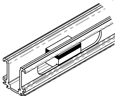
Kit distanziali vetro Kit glass spacer Kit distanciales para vidrio
