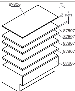
Spessori per vetro Glass thickness Espesores para vidrio
