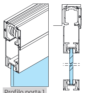
Profilo porta 1
